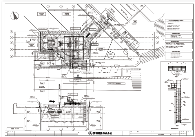
根伐計画図
