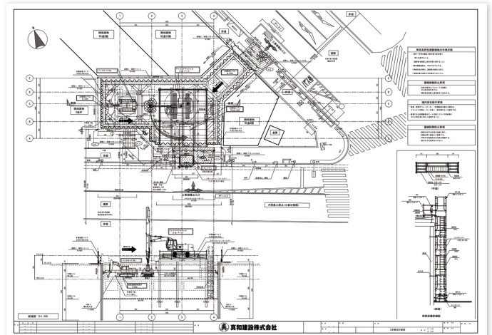
根伐計画図
