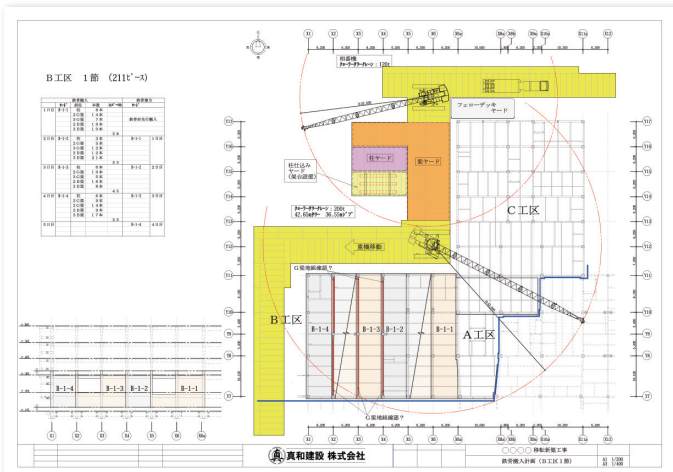
建方計画図
