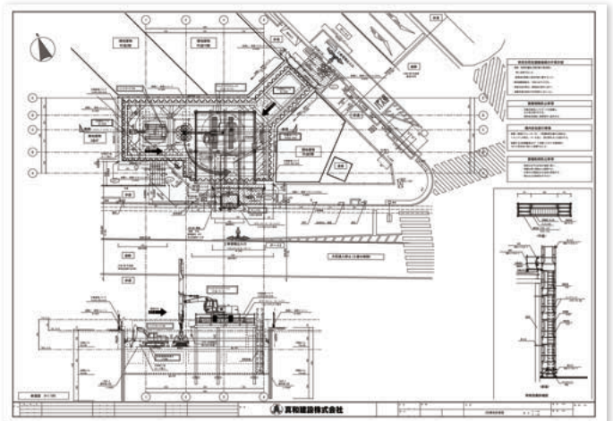
根伐計画図
